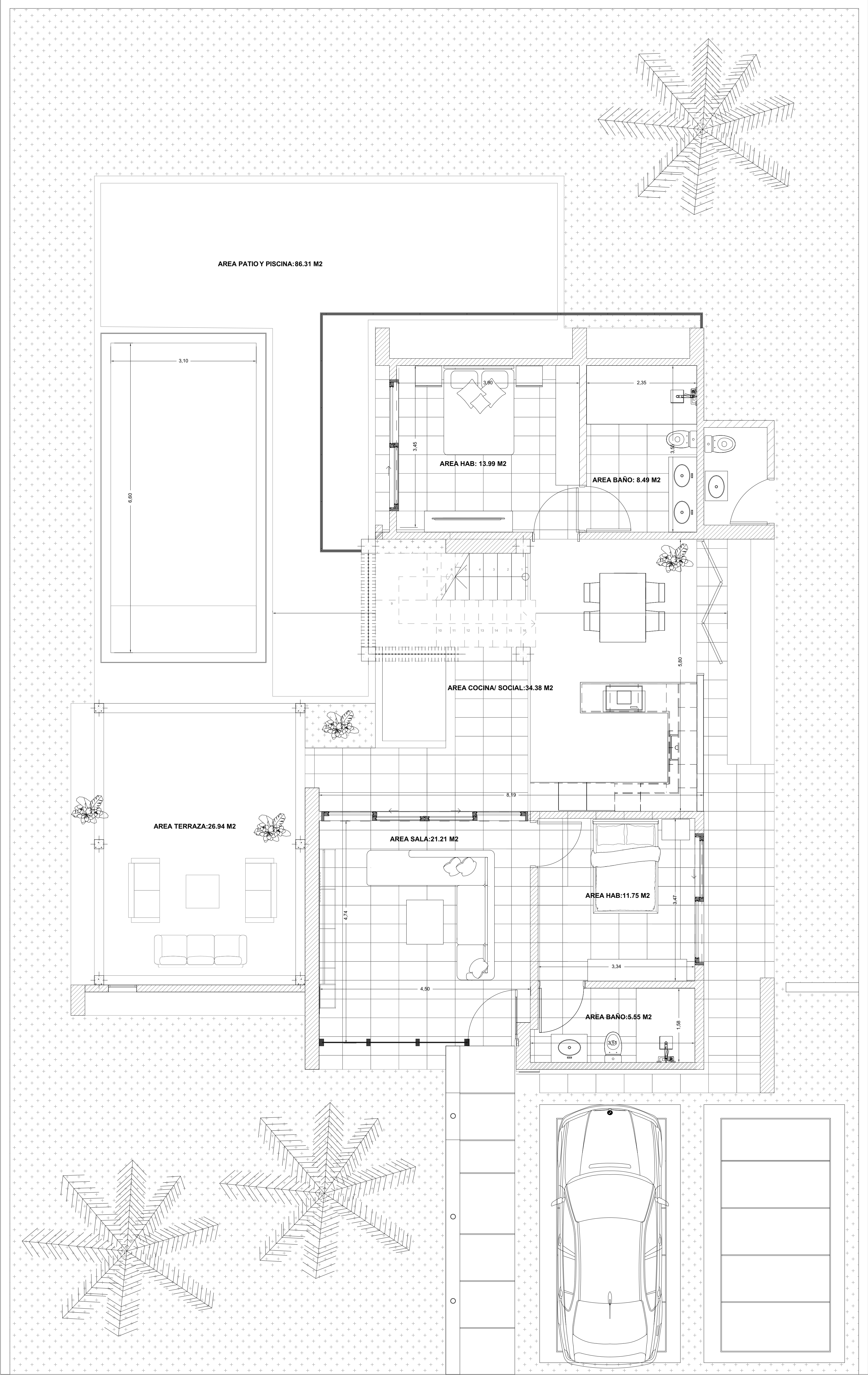
PLANTA ARQUITECTÓNICA PRIMER PISO CASA TIPO 3
